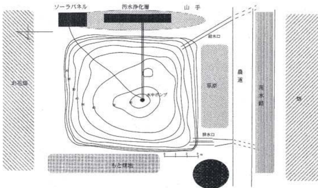
図1 1999年4月25日に改修されたニッポンバラタナゴの保護池(約140㎡)の水深(cm)と池周辺の状況。太陽電池と水中ポンプを利用した水浄化循環システムを2002年1月13日に設置した。
